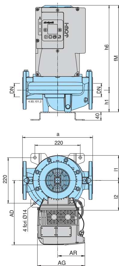
Flanges PN 10, EN 1092-2
